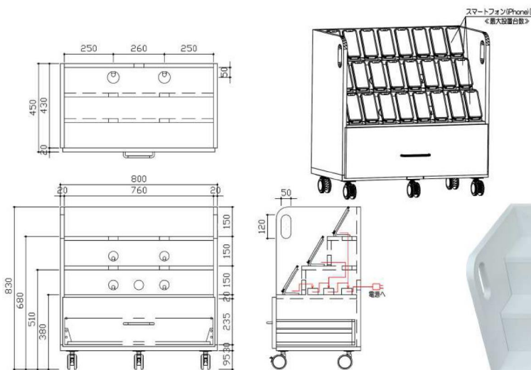
スマートフォン/iPhone(24台) 《最大設置台数》 スマートフォン/iPhone(24台) 《最大設置台数》 ※スマートフォンの機種に合わせて、 必要な台数の充電器を別途ご用意いたします。 詳しくは担当営業へご相談ください。
